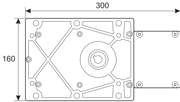
Блок подключения, вид сверху
